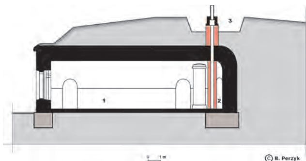
Przekrój pionowy koszar szyjowych: 1 – kazamata mieszkalna, 2 – korytarz wentylacyjno-grzewczy, 3 – reducja na linii ognia
