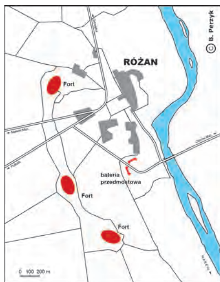
Pierwotny stan rozbudowy przedmościa Różana w roku 1888, w którym gotowa była pozycja złożona z dzieł fortyfikacji polowej
